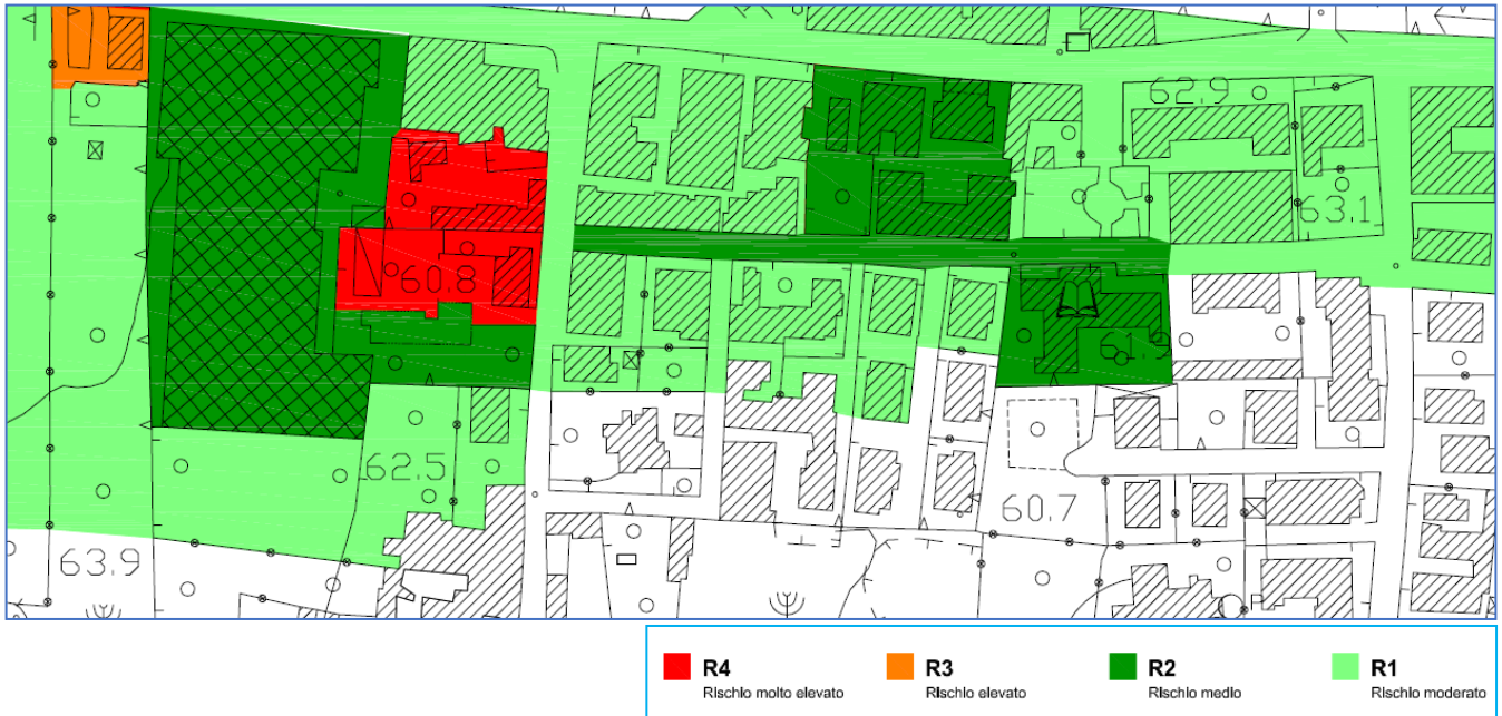
Comune di Nocera Superiore (SA) – torrente Cavaiola - Piano Stralcio di Assetto idrogeologico dell'ex AdB Campania Centrale – Stralcio mappa del rischio idraulica approvata (tav. 446081R)
